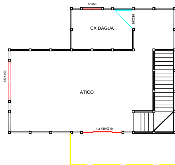
ÁTICO 42 MÓDULOS
