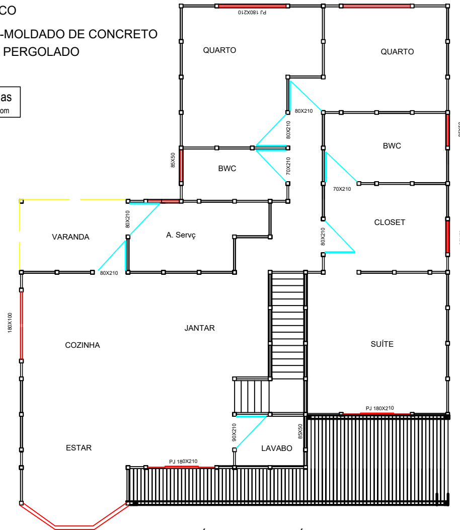
TÉRREO 123,75 MÓDULOS
